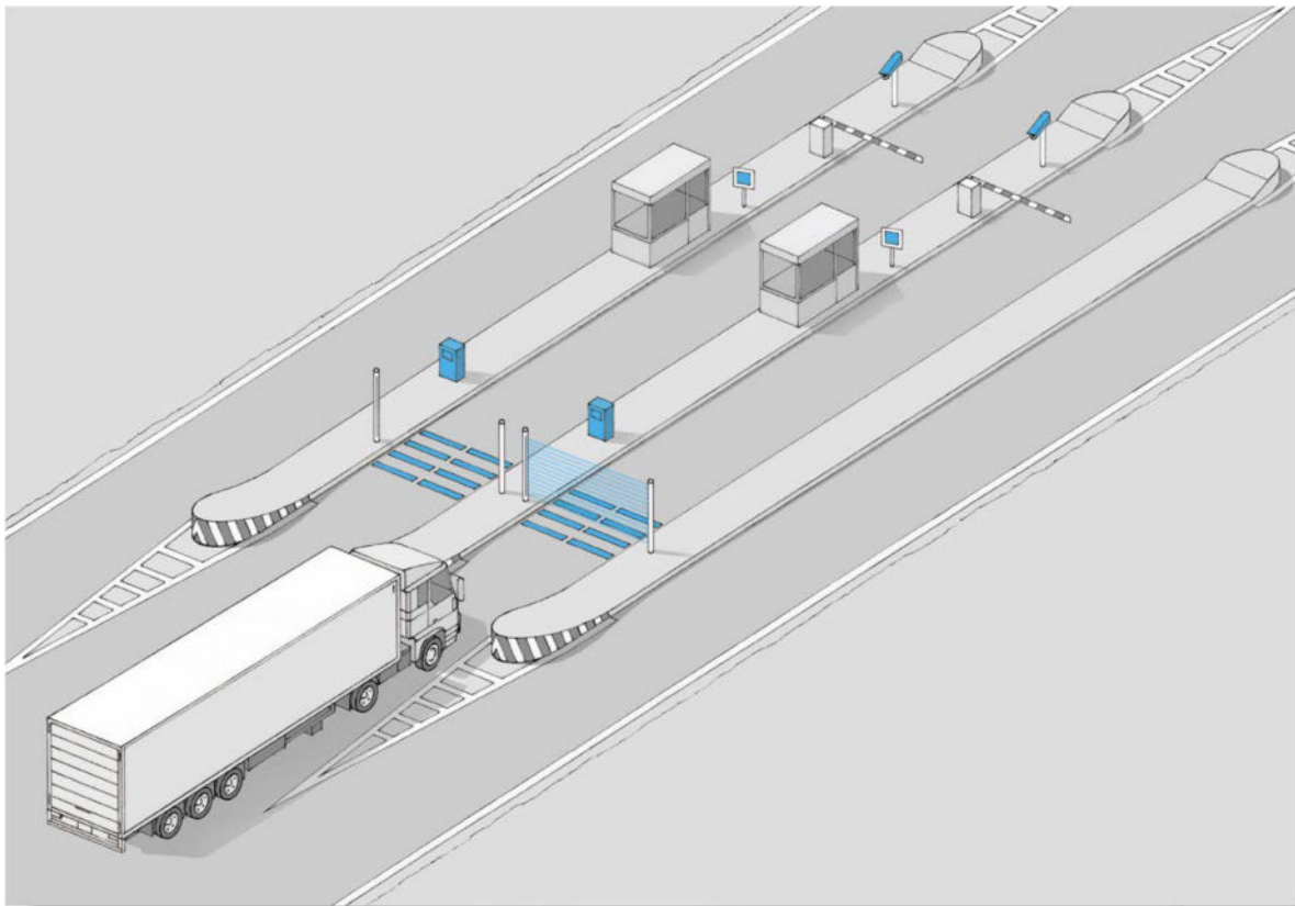
Schema di un tipico varco di pesatura
